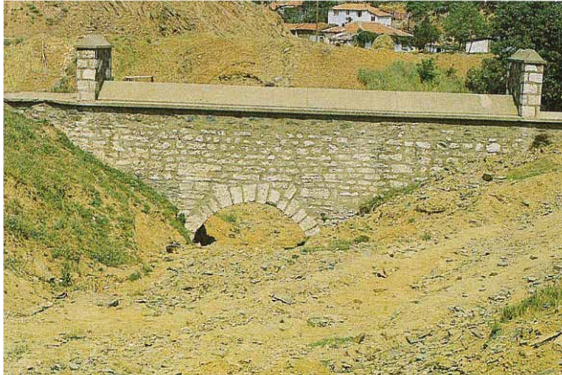
Resim 13: Dolap Kemerii I
