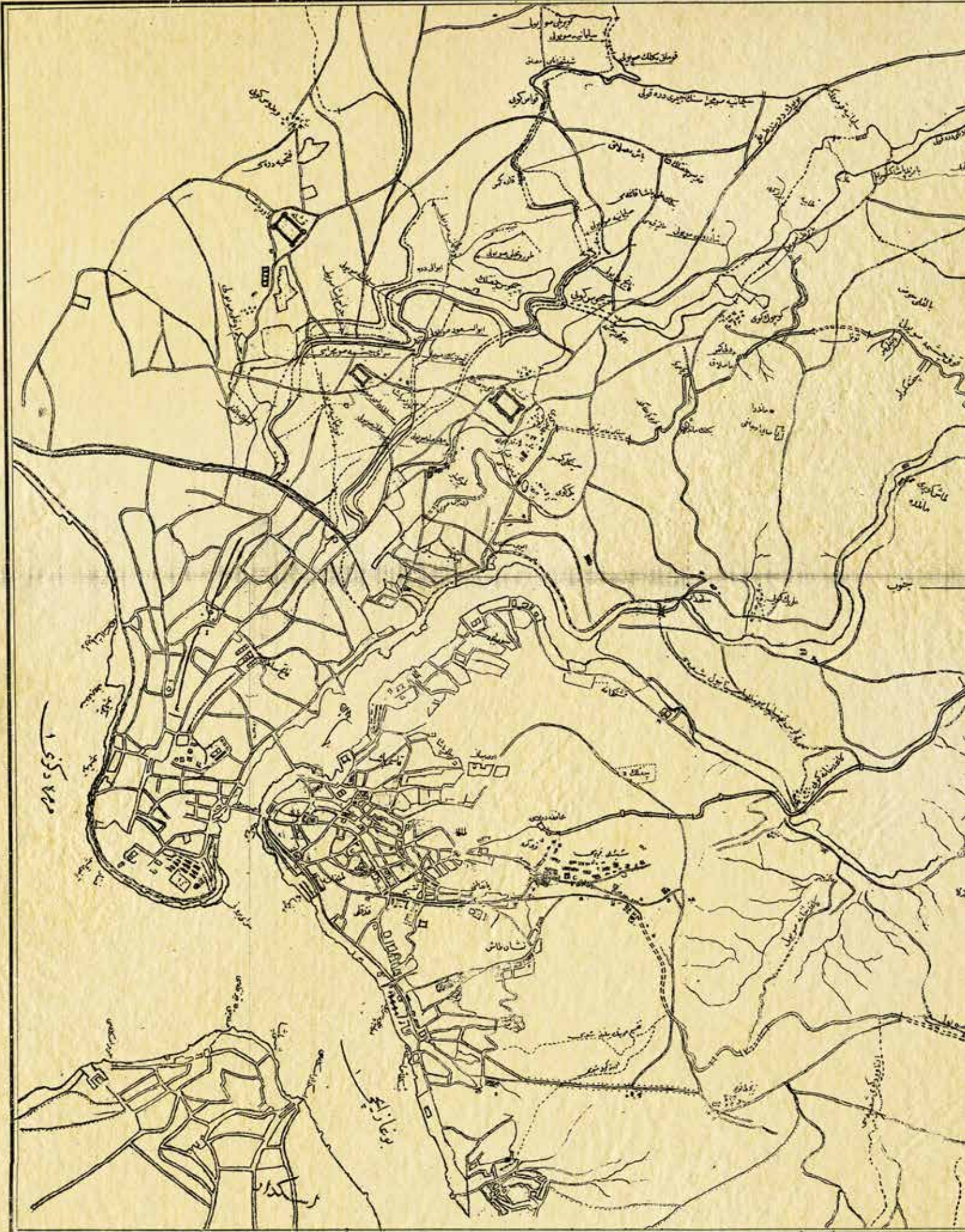
Harita 4: Kırkeçme, Taksim ve Halkalı Sularının Mebdelerile Şehir Haricindeki Mecralarını Gösterir Kroki
