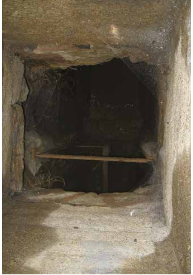
Resim 17: Tarihî Galeri Bacası I 16 (Keçesuyu tesisleri içerisinde)
